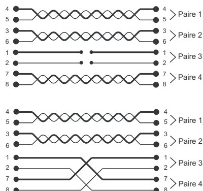
Ejemplos de esquemas de identificación de pares cortados y cruzados en los cables
